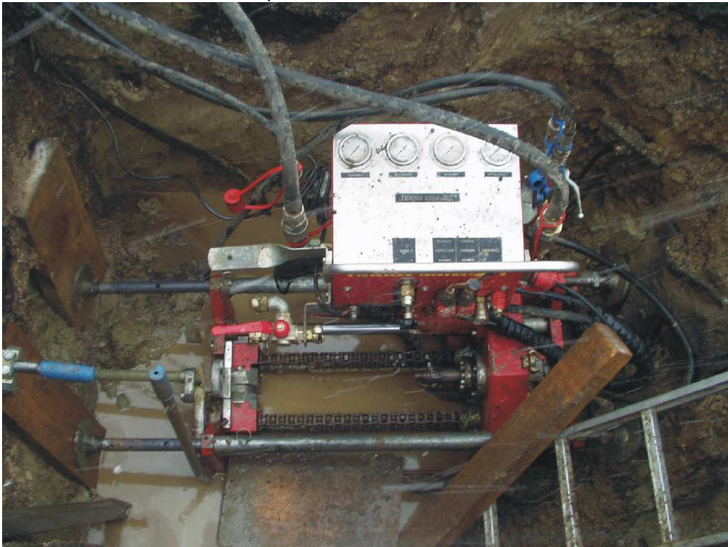
Установка TERRA MINI-JET в стартовом котловане.
