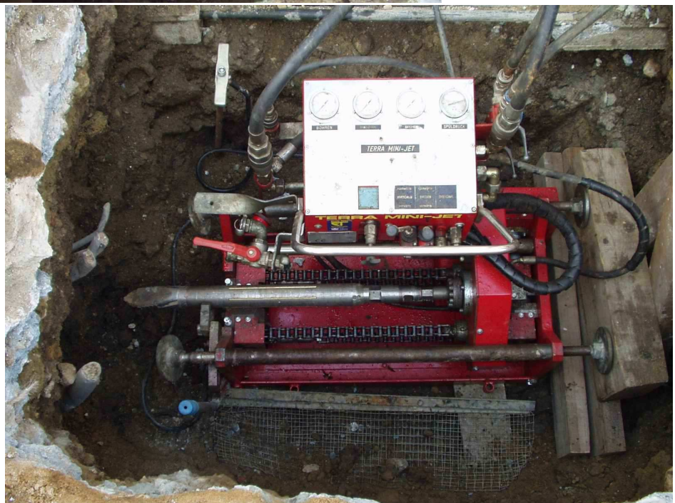
Фото справа: TERRA MINI-JET в стартовом котловане перед началом пилотного бурения.
